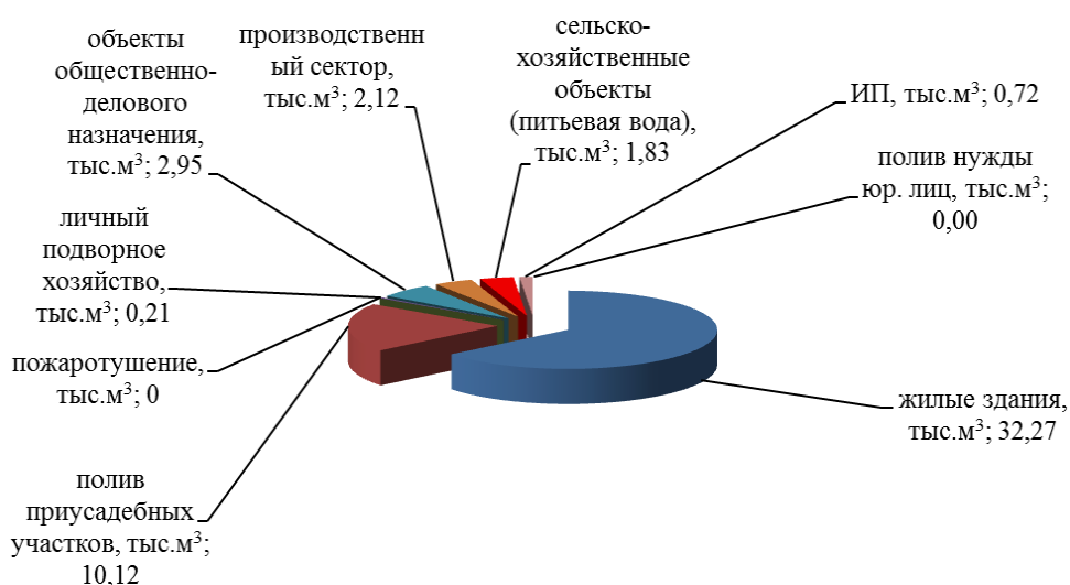
Рисунок 12 – Развернутый годовой структурный баланс реализации питьевой воды
