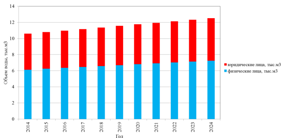
Рисунок 28 – Перспективный структурный баланс горячего водоснабжения
