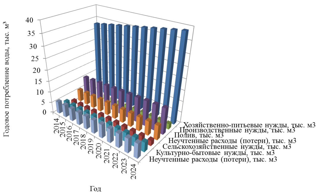
Рисунок 16 – Прогнозные балансы потребления питьевой воды до 2024 г.
