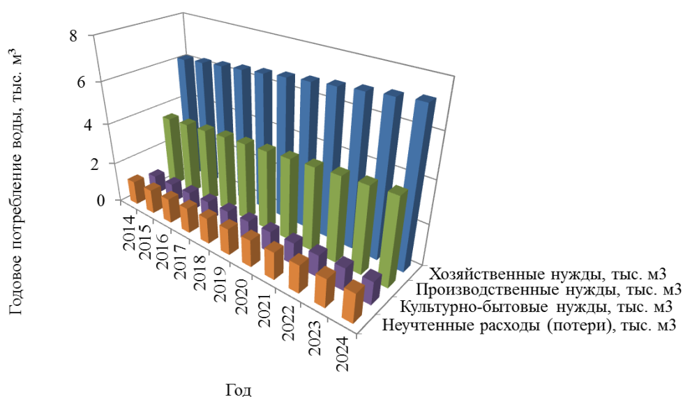
Рисунок 17 – Прогнозные балансы потребления горячей воды до 2024 г
