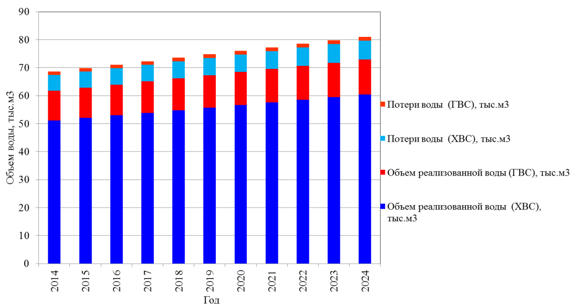
Рисунок 25 – Перспективный общий баланс подачи и реализации водоснабжения
