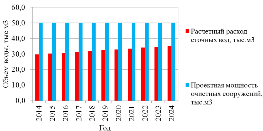
Рисунок 32 – Соотношение существующего и перспективного расхода сточных вод и мощности очистных сооружений пос. Озерный
