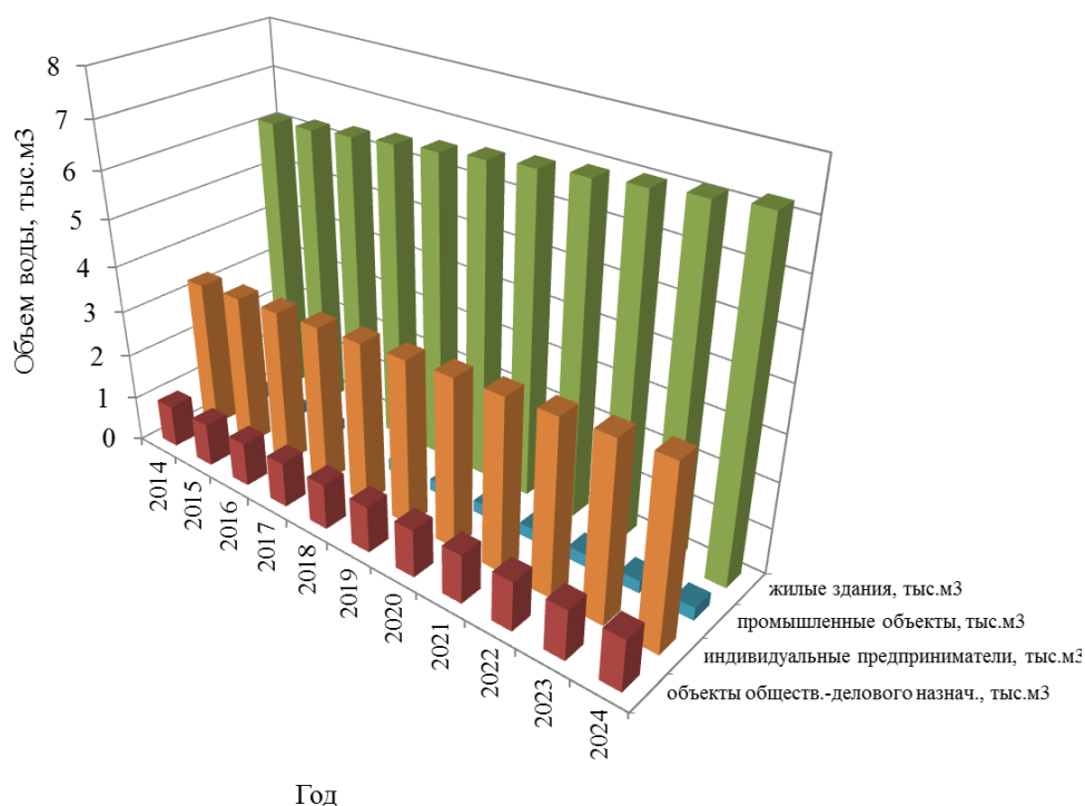
Рисунок 22 – Прогноз распределения расходов воды на водоснабжение по типам абонентов
