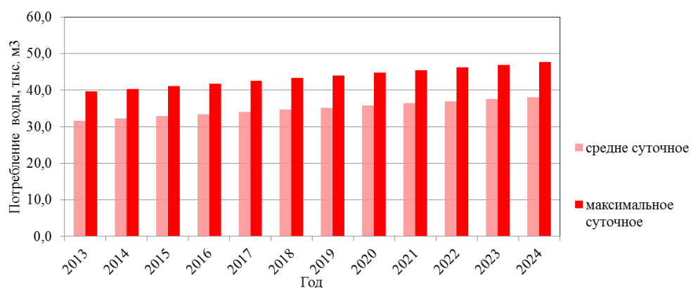
Рисунок 20 – Фактическое и ожидаемое среднесуточное и максимальное потребление горячей воды
