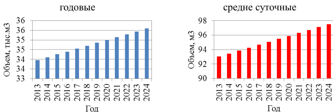
Рисунок 23 – Сведения о годовых фактических и планируемых потерях питьевой воды при ее транспортировке
