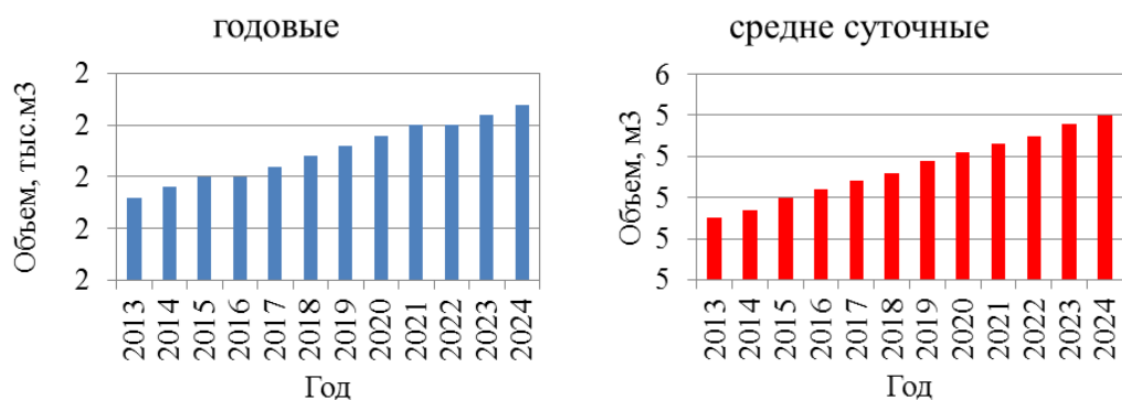
Рисунок 24 – Сведения о годовых фактических и планируемых потерях горячей воды при ее транспортировке
