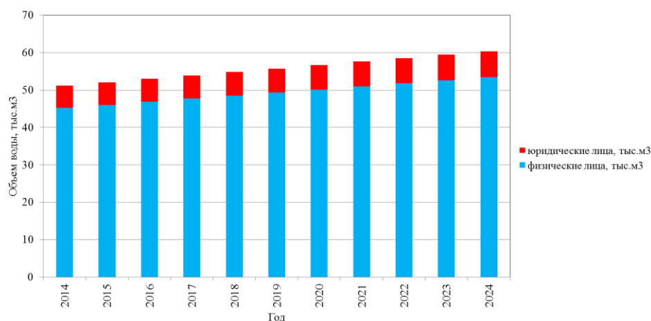
Рисунок 27 – Перспективный структурный баланс водоснабжения
