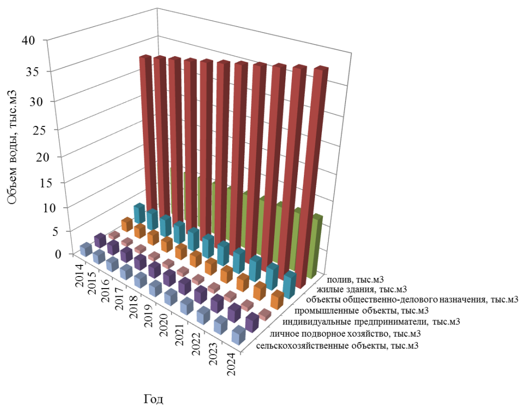
Рисунок 21 – Прогноз распределения расходов воды на водоснабжение по типам абонентов
