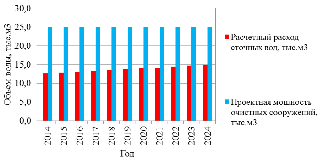
Рисунок 31 – Соотношение существующего и перспективного расхода сточных вод и мощности очистных сооружений д.п. Мочище
