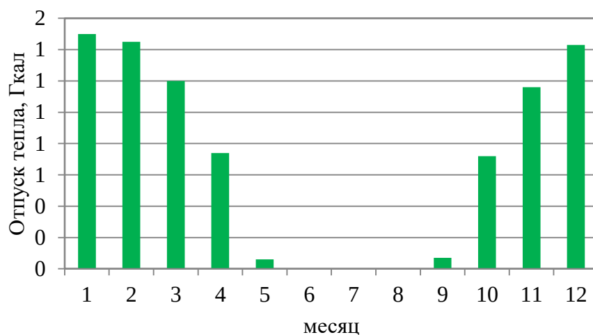
Рисунок 1.12 – Оптимальный температурный график отпуска тепловой энергии для котельной ул. Нагорная, 32 д.п. Мочище
