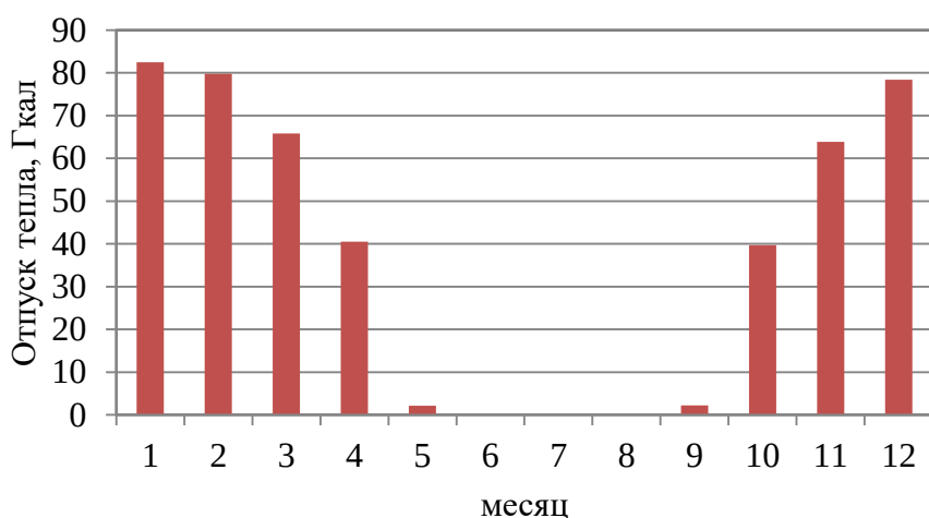
Рисунок 1.13 – Оптимальный температурный график отпуска тепловой энергии для котельной СОШ №45 д.п. Мочище
