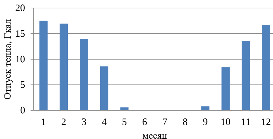
Рисунок 1.15 – Оптимальный температурный график отпуса тепловой энергии для котельной в ул. Первомайская, 242А д.п. Мочище
