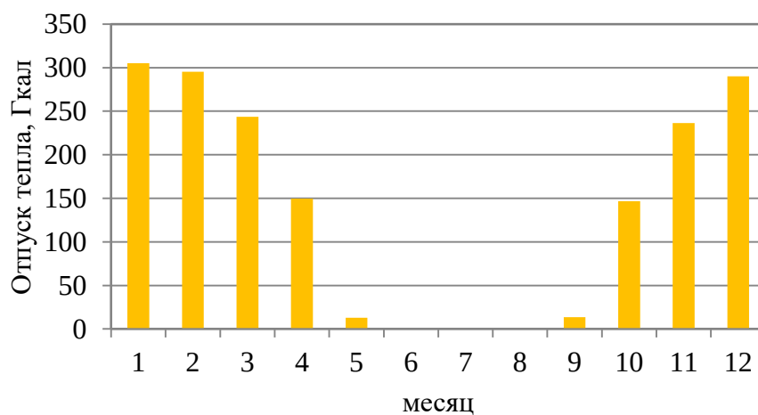
Рисунок 1.14 – Оптимальный температурный график отпуска тепловой энергии для котельной в ул. Набережная, 1А д.п. Мочище
