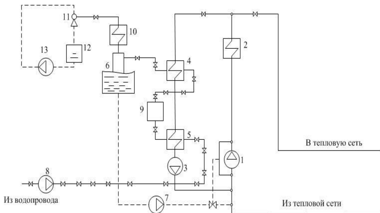
Рисунок 2.6 – Принципиальная тепловая схема котельной с водогрейными котлами:
