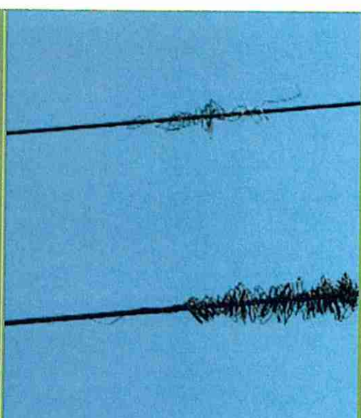
Поврежденный провод ВЛ 110 кВ
